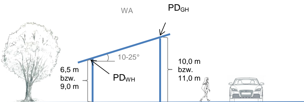
Abbildung 8: Prinzipskizze für Gebäude mit Pultdach
